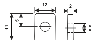
БОЛТ И ГАЙКА М5
